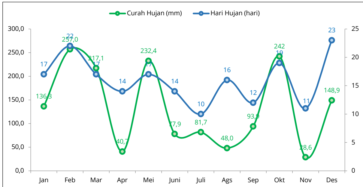
Gambar 1.2 Curah Hujan dan Banyak hari Hujan di Banyuwangi Tahun 2020
