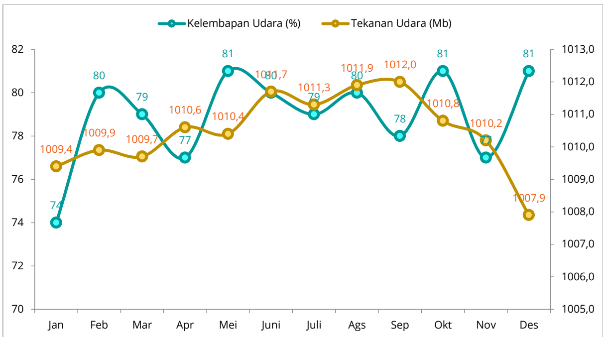
Gambar 1.4 Kelembapan dan Tekanan Udara di Banyuwangi Tahun 2020
