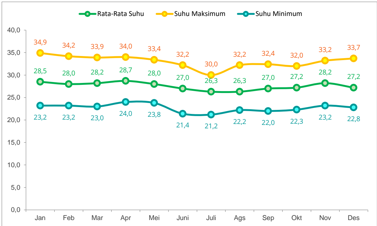
Gambar 1.3 Suhu Rata-rata, Suhu Minimum dan Maksimum di Banyuwangi Tahun 2020
